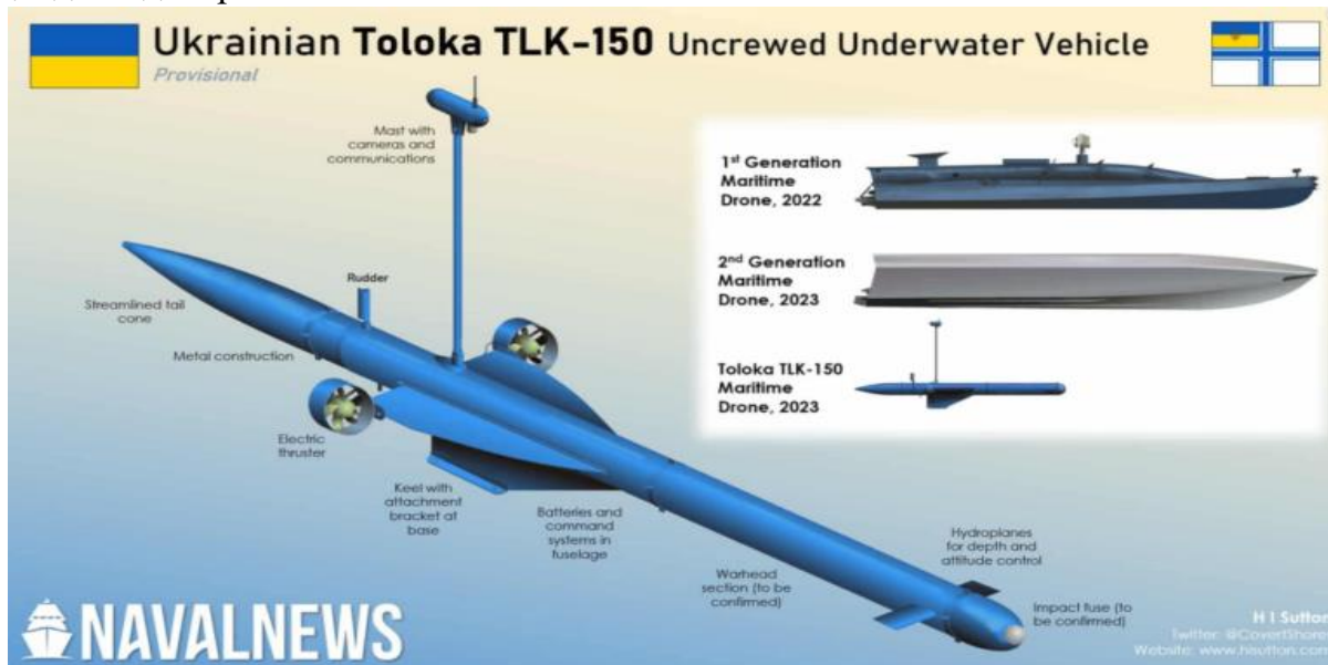
Вигляд українського підводного морського дрона Толока Т-150. Джерело NAVALNEWS.
