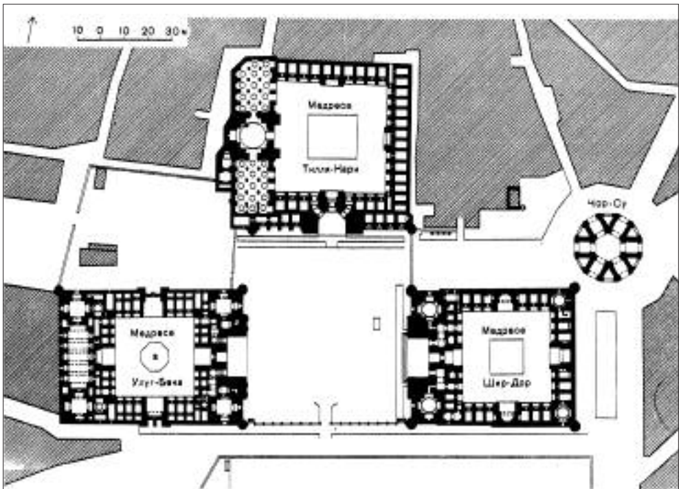
План ансамблю Регістан у Самарканді
