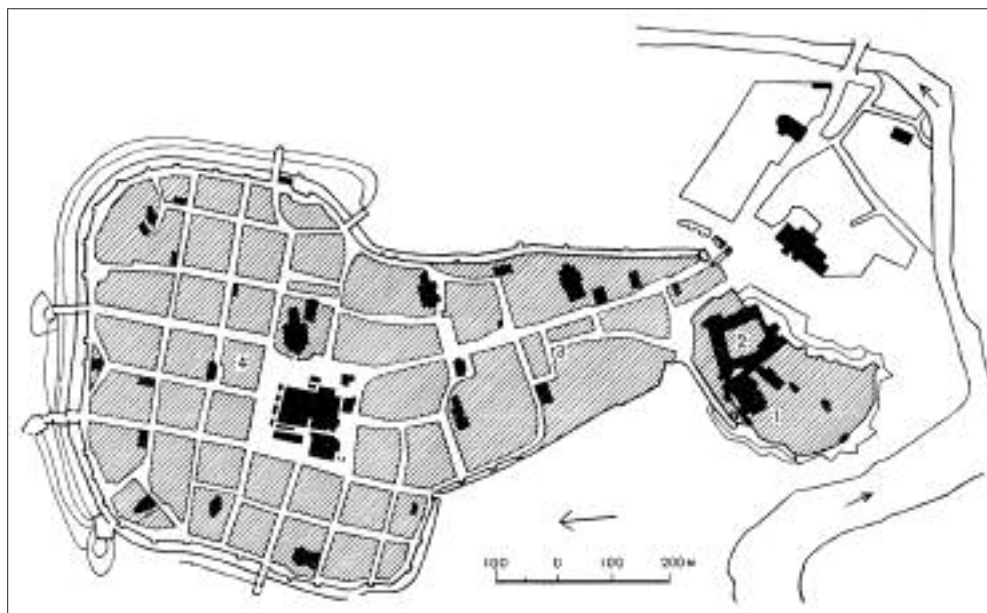
План середньовічного Кракова:
