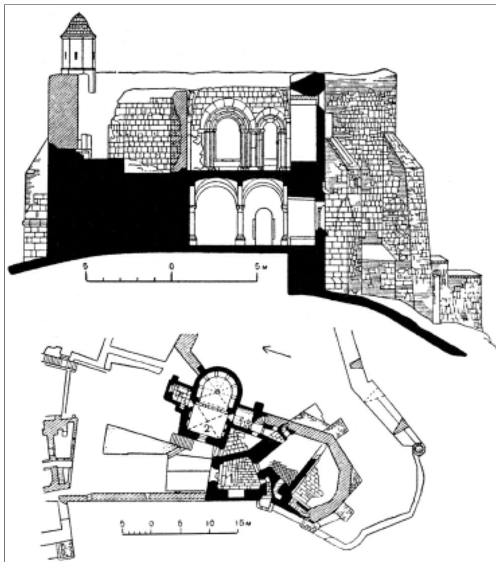
Королівський замок в Естергомі, розріз і план: 1 – тронний зал; 2 – капела
