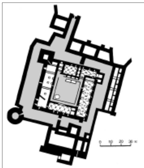
План орденського замку в Вільянді
