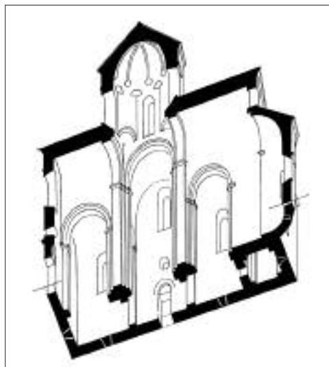
Аксометричний розріз церкви в Мрені
