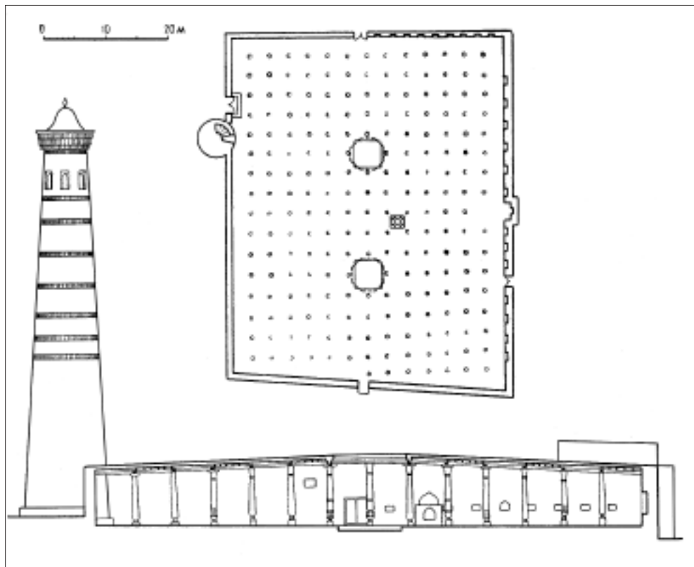
План і розріз соборної мечеті в Хіві
