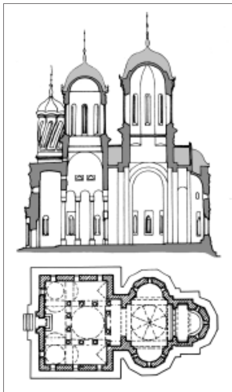
Єпископська церква—усипальниця в Куртя де Арджеш. План і поздовжній розріз
