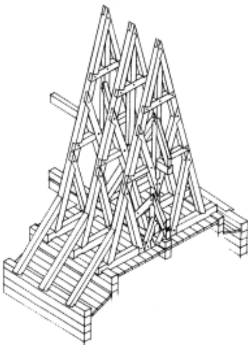
Дерев'яна конструкція даху готичного костелу
