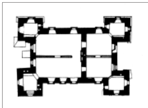
План замку в Баранові
