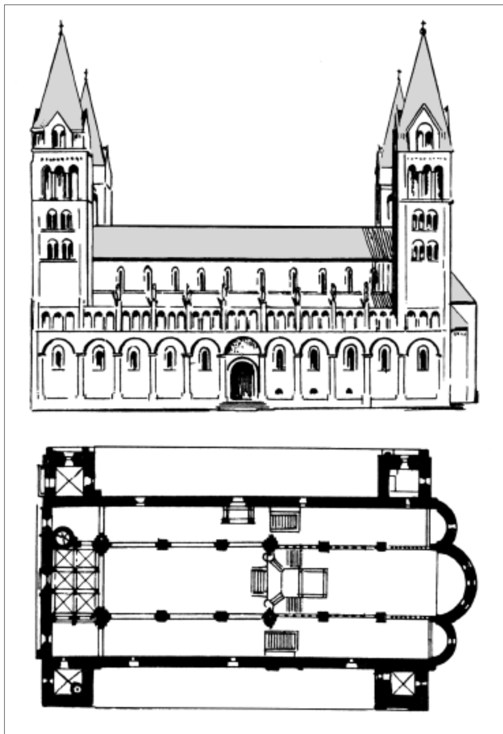
Собор у місті Печ. Південний фасад і план
