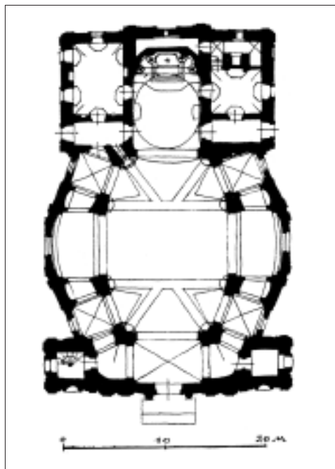
План костелу Св. Анни в Любартові
