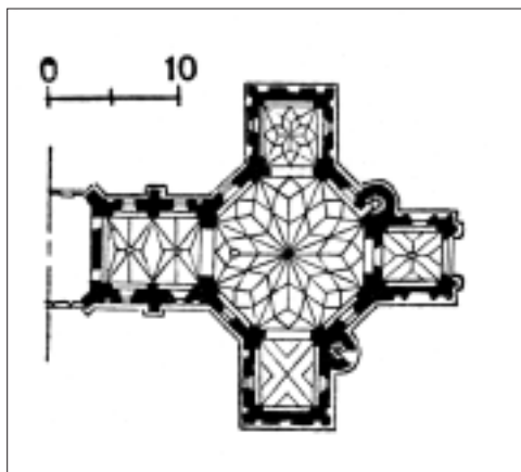
План церкви в Гославицях
