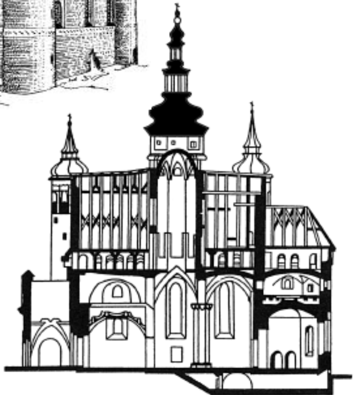
Благовіщенська церква у Супраслі. Поздовжній розріз
