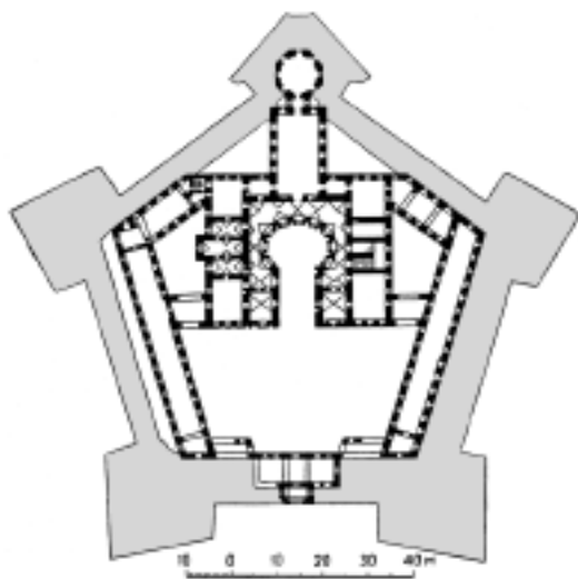
План замку в Кшиштопорі
