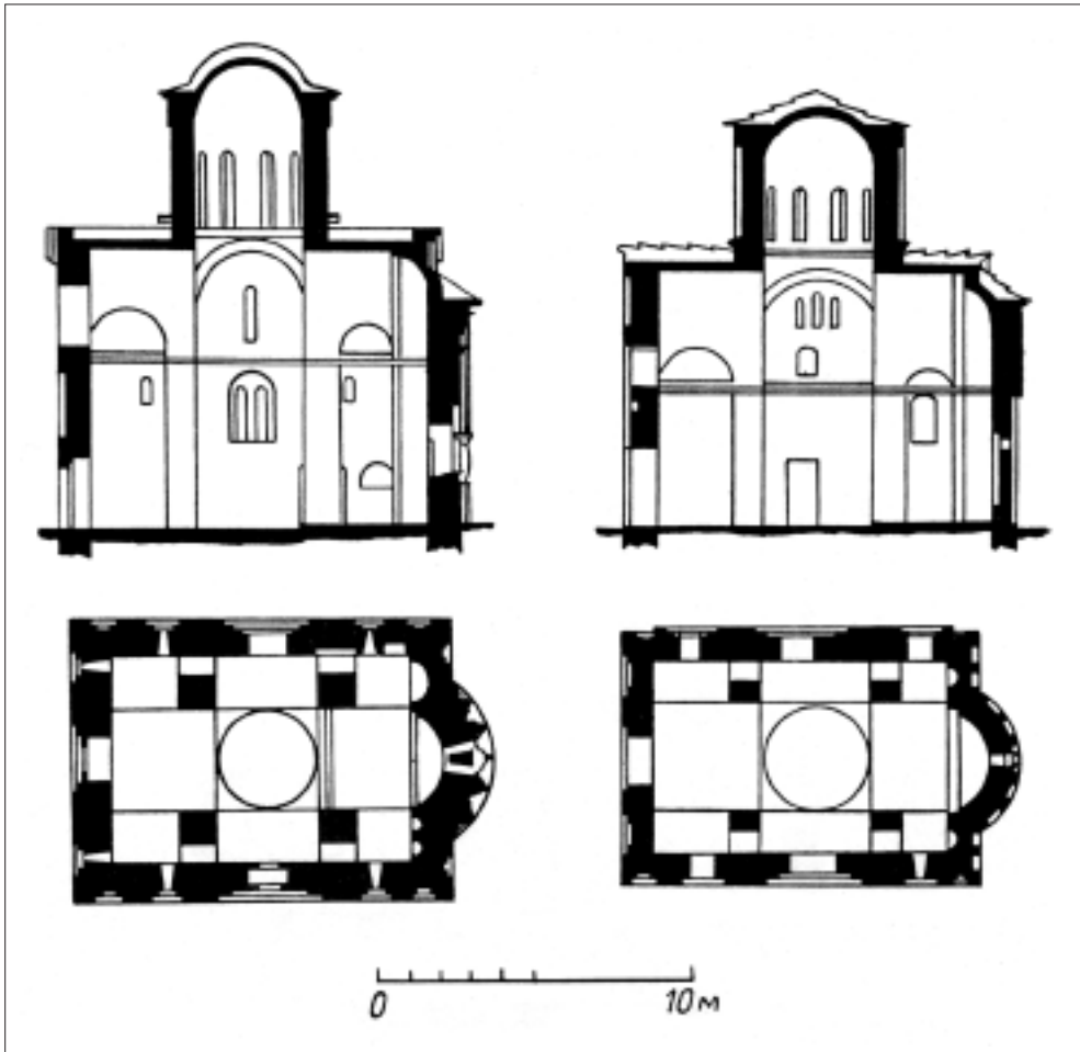
Плани й поздовжні розрізи церков Македонської і Косовсько—Метохійської школи: Архангелів у монастирі Лісново; Архангелів у Штіні
