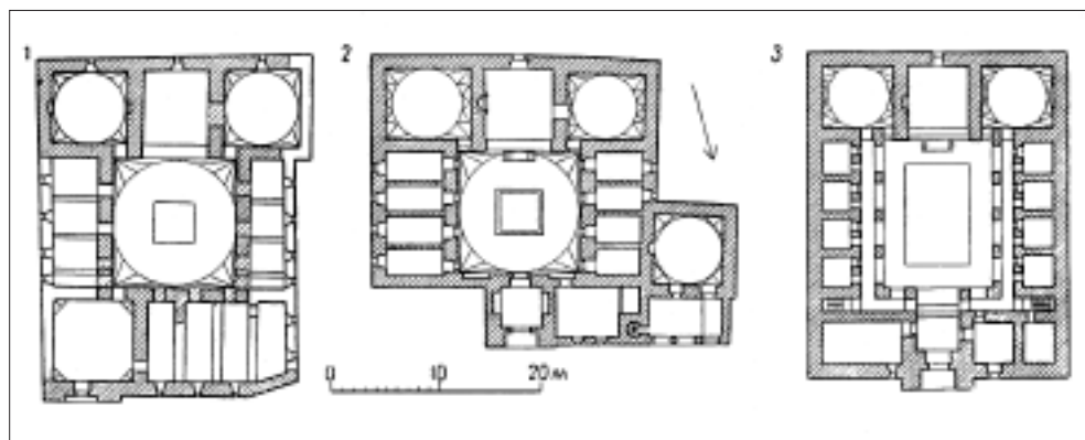
Плани сельджуцьких медресе XIII ст. у Кон'я:
