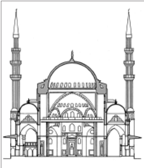
Поперечний розріз мечеті Сулейманіє в Стамбулі
