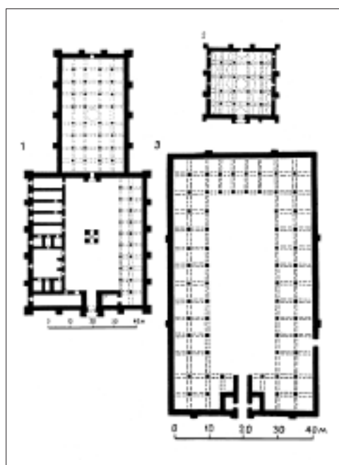
Плани ханів сельджуцького періоду:
