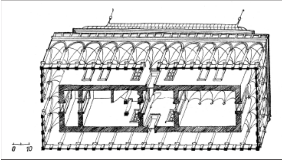
Бельведер у Празі. Аксонометричний розріз
