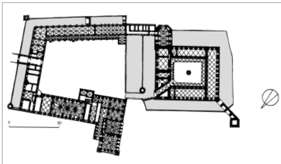
План центральної частини замкового ансамблю в Марієнбурзі
