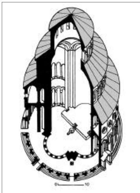
Аксометричний розріз храму Звартноц за реконструкцією Т. Тораманяна
