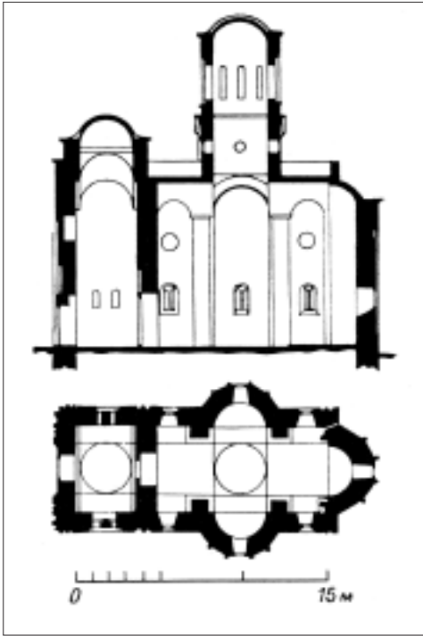
Церква монастиря Каленич. План і поздовжній розріз
