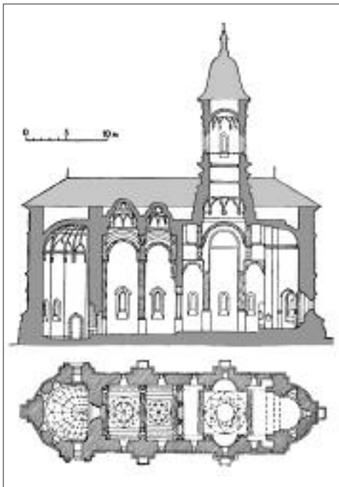
Церква монастиря Драгомирна. Поздовжній розріз і план
