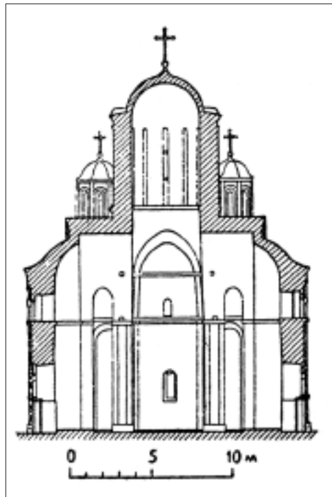
Розріз церкви в Раваниці
