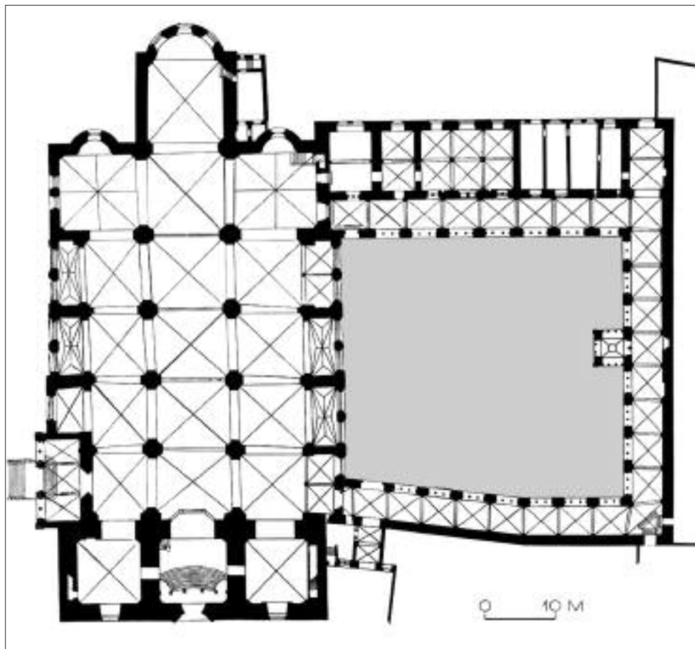
План ансамблю Домського собору в Ризі
