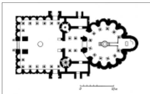
План Круглої церкви в Преславі
