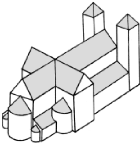
Схема об'ємно—просторової композиції костелу в Кружвиці
