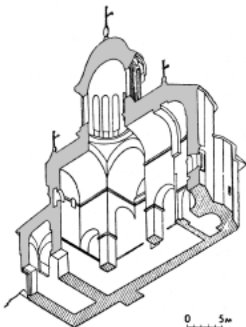
Церква Св. Миколая в Куртія де Арджеш. Аксонетричний розріз
