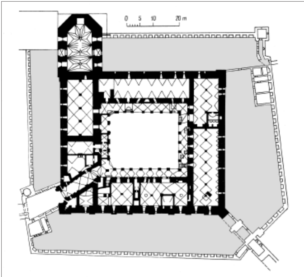
План Високого замку в Марієнбурзі
