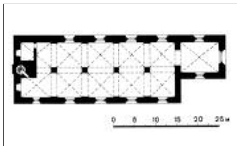
План церкви Св. Духа в Таллінні
