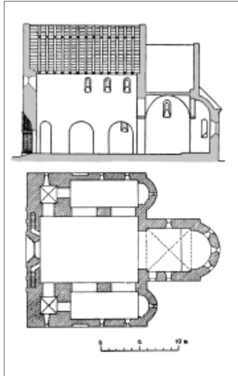
Церква в Чиснедоарі. Поздовжній розріз і план
