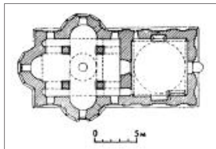
План церкви в Любостині
