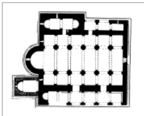
План базилики Сіоні в Болнісі
