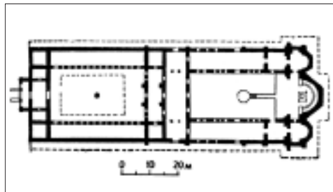
План «Великої базиліки» в Плиссі
