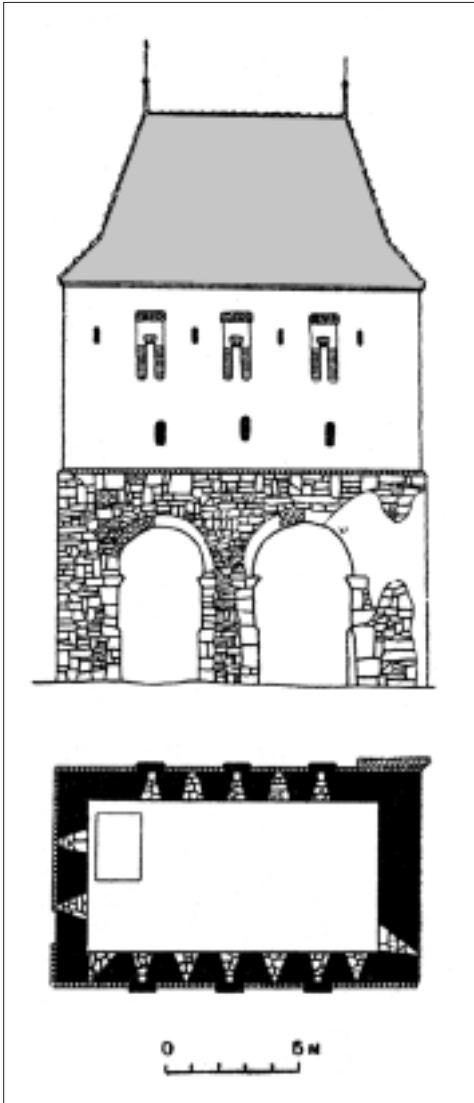
Кравецька надбрамна башта міських мурів Сігішоарі. Фасад і план третього ярусу
