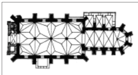
План костелу у Вислиці
