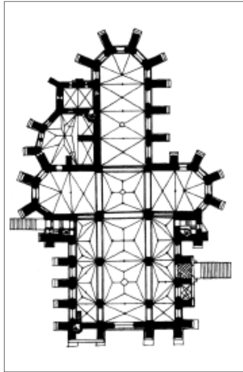
План костелу Св. Хреста у Вроцлаві
