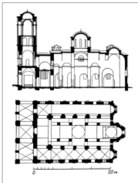
Церква Левиської Богородиці в Призрені. План і поздовжній розріз
