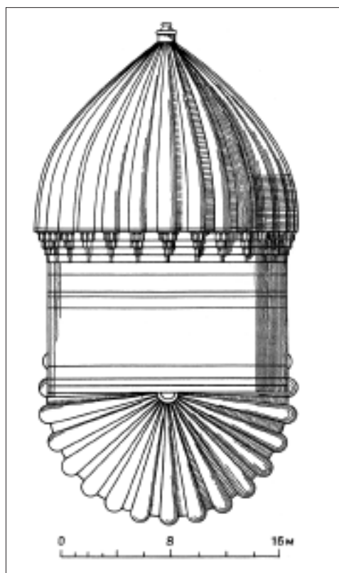
Гофрований (складчастий) купол медресе Шир-Дор у Самарканді
