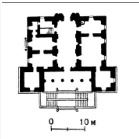
План вілли у Волі Юстовській
