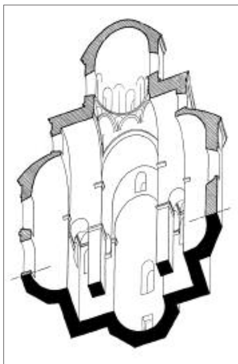
Церква Теодороса в Багарані. Аксометричний розріз
