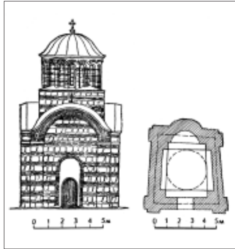
Церква у Діноджеїї. Фасад і план
