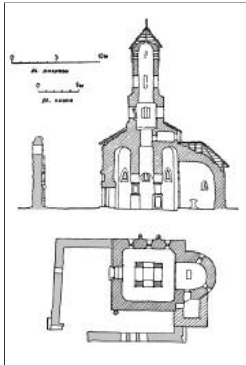
Церква в Денсуші. Поздовжній розріз і план
