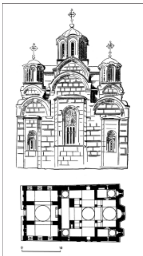
Церква в Грачаниці. Східний фасад і план
